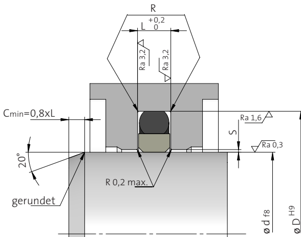
Einbauräume nach ISO 7425/2
